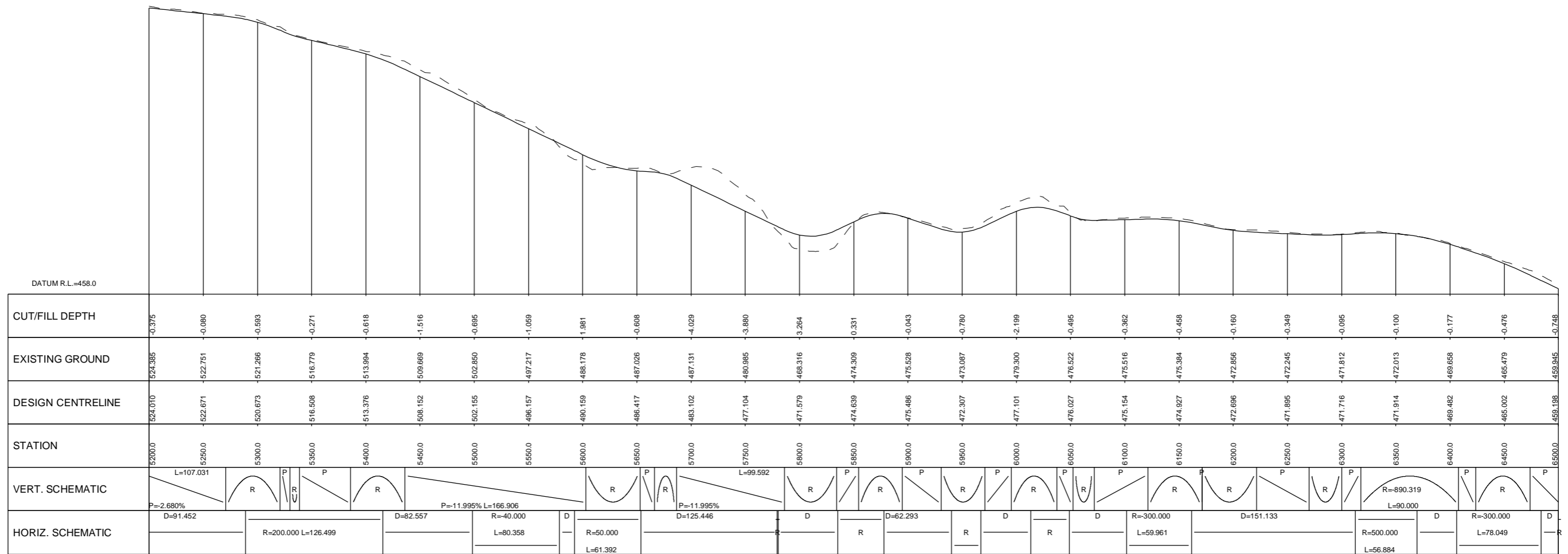
LONG SECTION SCALE 1 : 2000 Hz 1 : 500 Vt
